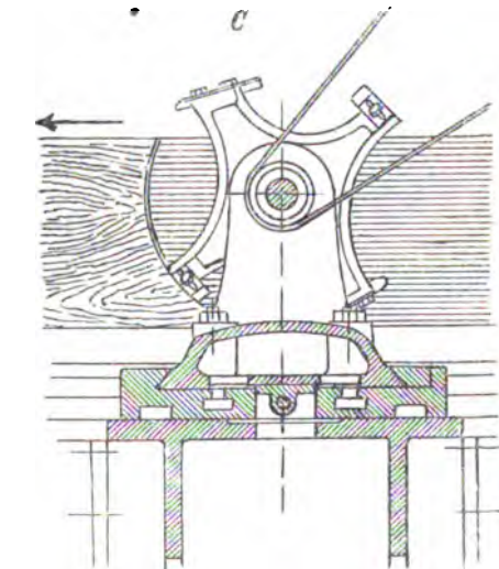
C. 1732. Hoblovací stroj na dřevo (uspořádání nožů).
